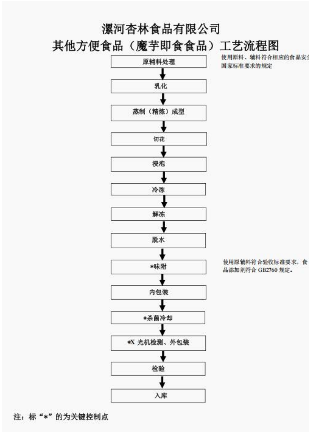
图 3-2 产品生产工艺流程图
